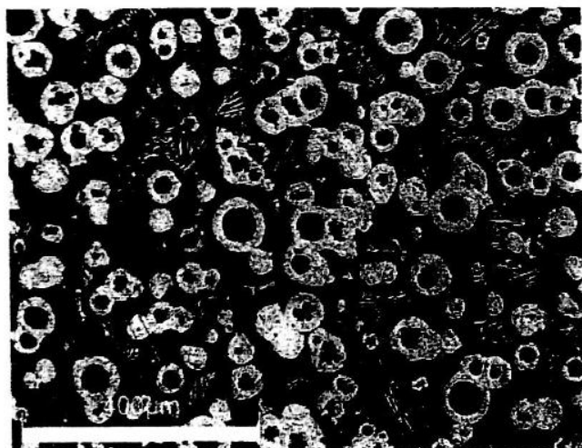
รูปที่ 2 โครงสร้างทางจุลภาคหลังการกัดกรด (Nitral 2%) พบกราฟไฟต์ชนิดก้อนกลมกระจายตัวอยู่ในชิ้นงาน โดยมีโครงสร้างพื้นฐานหลักเป็นโครงสร้างเพอริไรท์ โครงสร้างเฟอไรต์และมีโครงสร้างคาร์ไบด์ปรากฏอยู่
