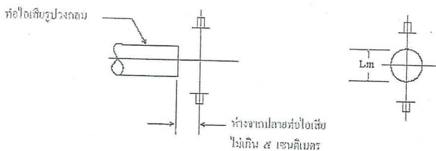
ภาพที่ ๑ สำหรับท่อไอเสียวงกลมชนิดตรง
